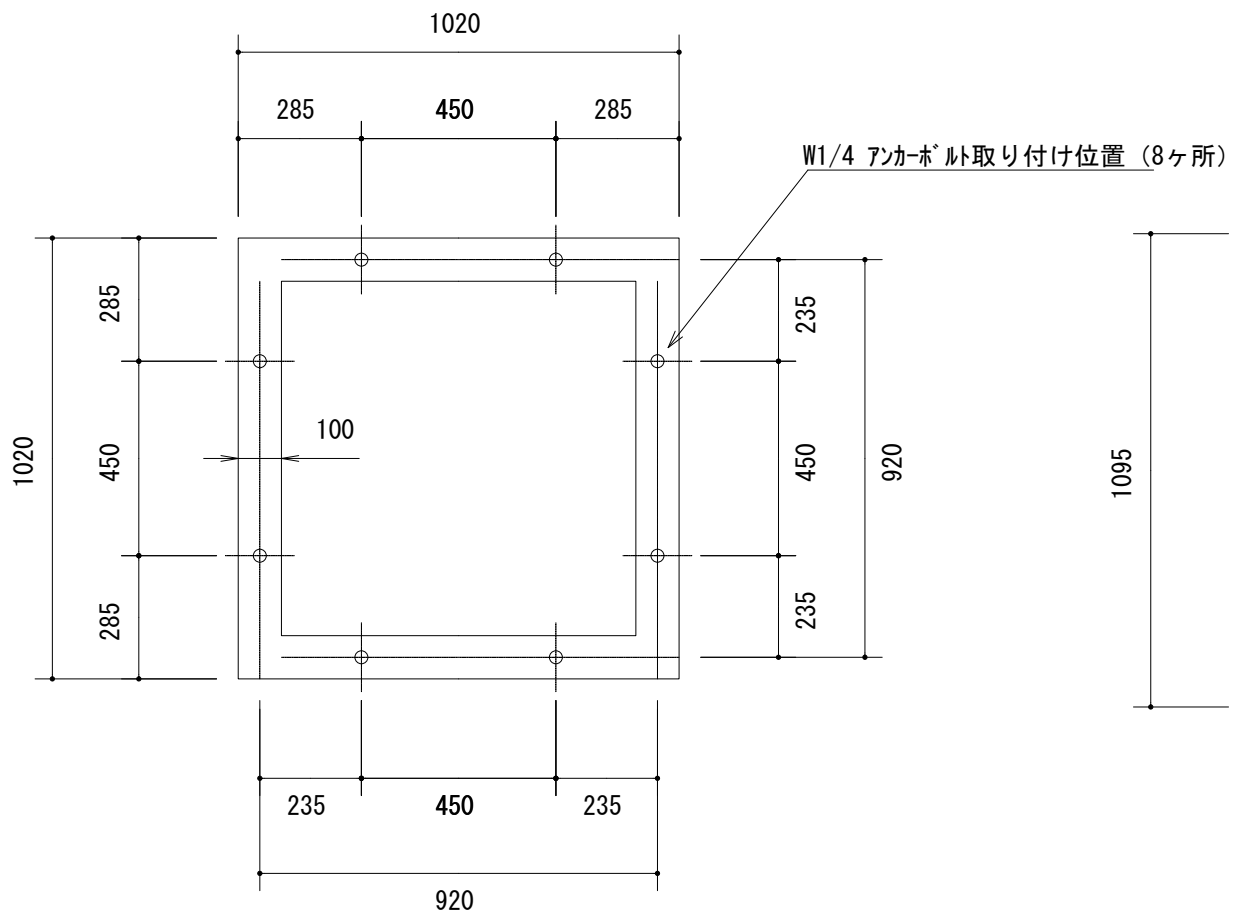
基礎図
