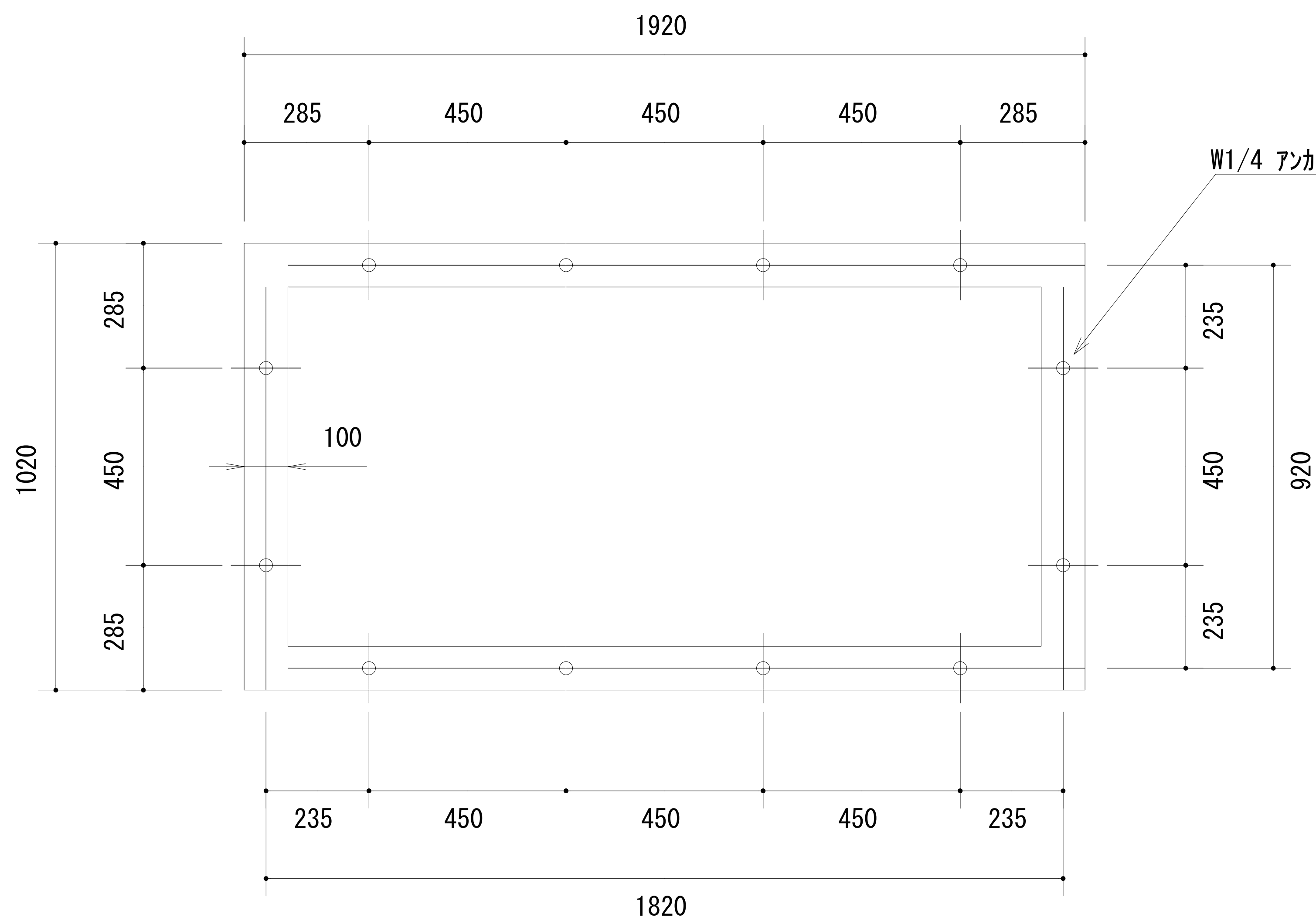
基礎図
